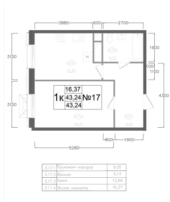
План типового 4-11 этажа Корпус 1 Секция 3 Квартира №17
