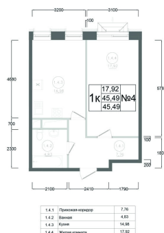
План типового 12-15 этажа Корпус 1 Секция 1 Квартира №4
