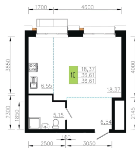
План 2 этажа Корпус 1 Секция 1 квартира №5
