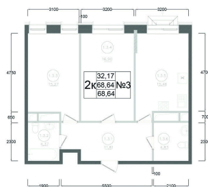
План 2 этажа Корпус 1 Секция 1 Квартира №3
