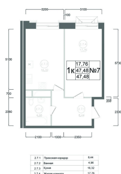
План типового 4-11 этажа Корпус 1 Секция 2 Квартира №7
