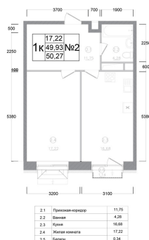
План 2 этажа Корпус 2 Квартира №2
