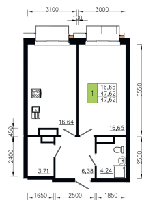
План 21 этажа Корпус 1 Секция 3 квартира №7
