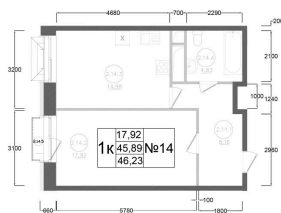
План 3 этажа Корпус 1 Секция 2 Квартира №14
