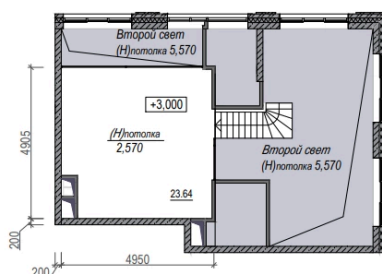
План антресоли
