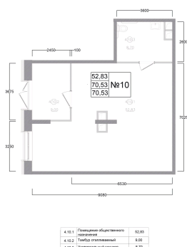
План 1 этажа Корпус 1 Секция 4 Офис №10
